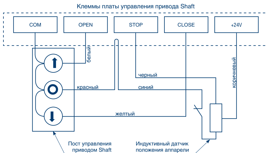
Рис. 5.2. Схема подключения индуктивного датчика положения аппарели*
