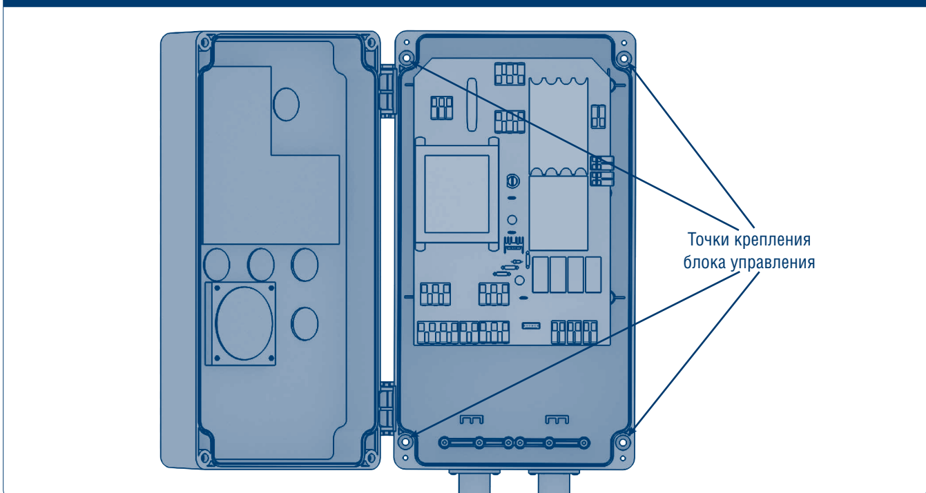
Рис. 4.1. Точки крепления блока управления
