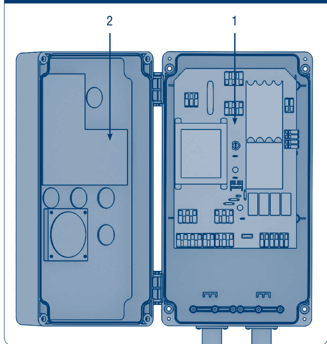
Рис. 3.2. Открытое положение блока управления
